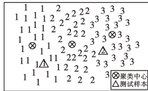
图1 改进算法中测试样本选择训练样本集的过程
